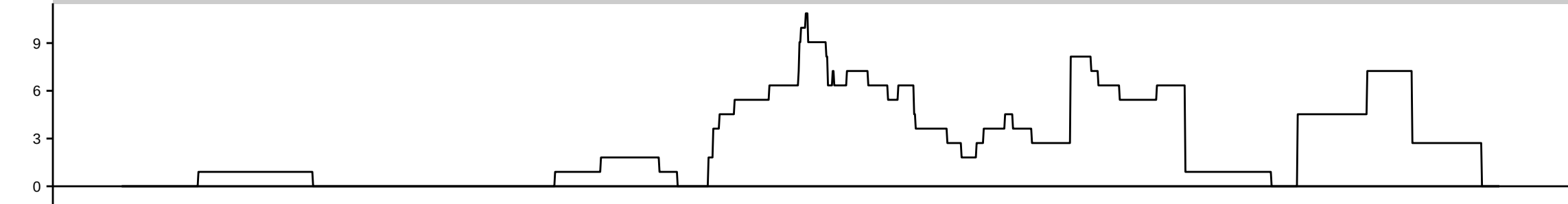
HsBam_polyA_whiteKD_00h_A
