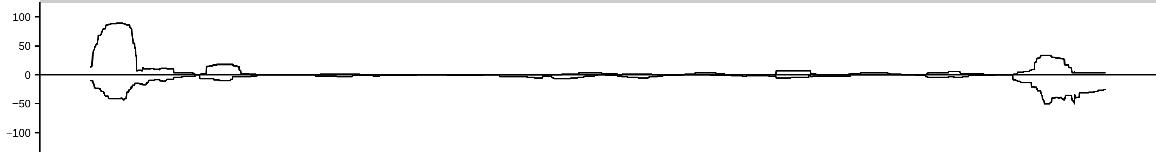
HsBam_polyA_whiteKD_00h_B
