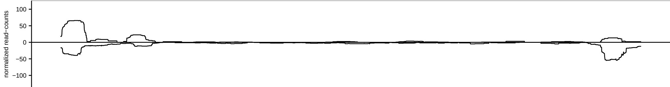
HsBam_polyA_whiteKD_00h_B
