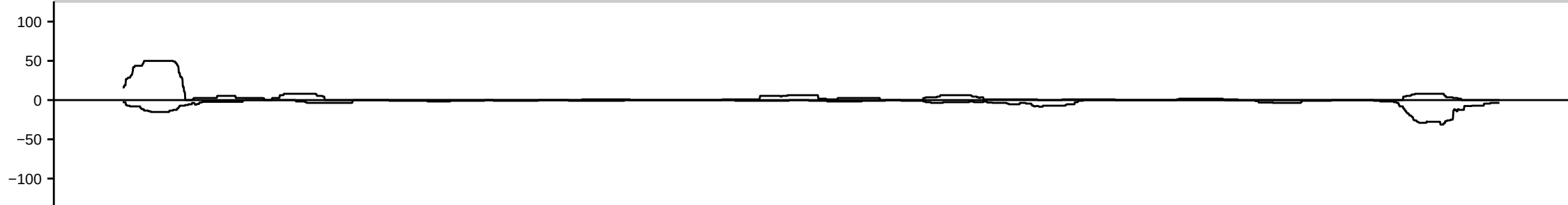
OV_polyA_piwiKD_B
