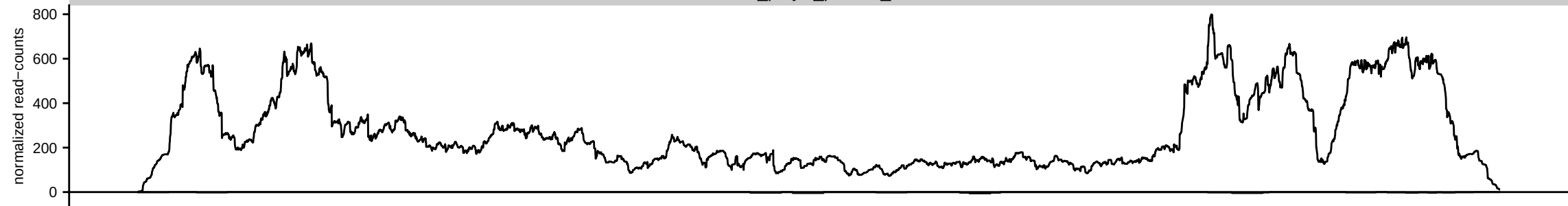
OV_polyA_piwiKD_B
