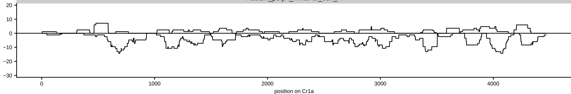
HsBam_polyA_whiteKD_68h_A
