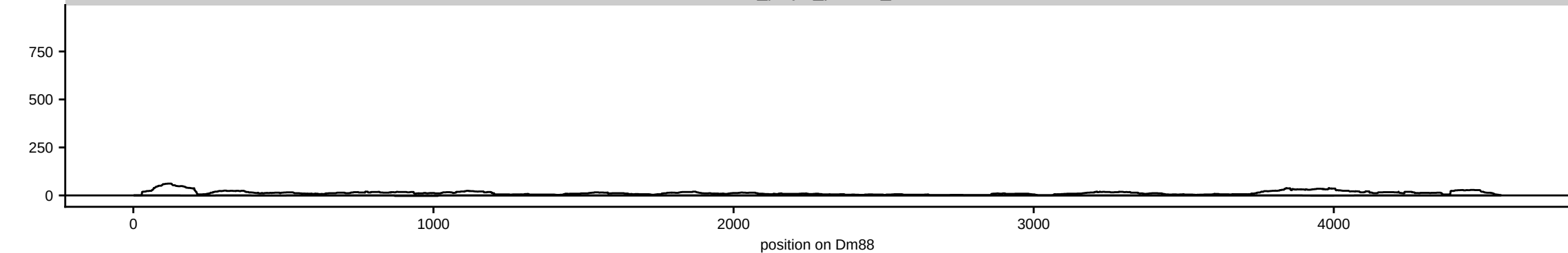
OV_polyA_piwiKD_B
