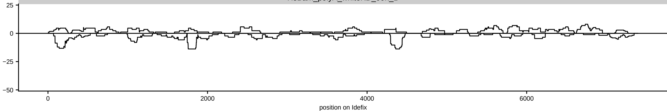
HsBam_polyA_whiteKD_00h_B
