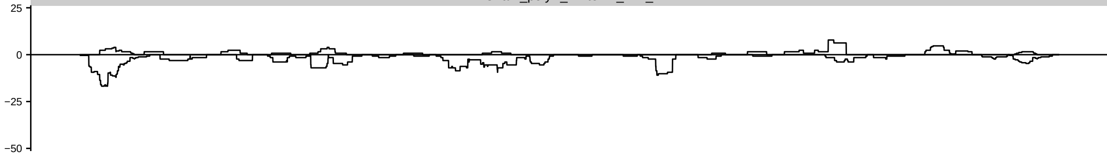
HsBam_polyA_whiteKD_42h_B
