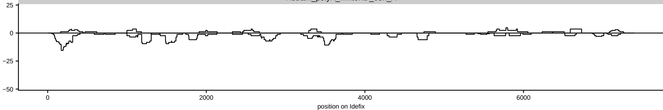
HsBam_polyA_whiteKD_68h_A
