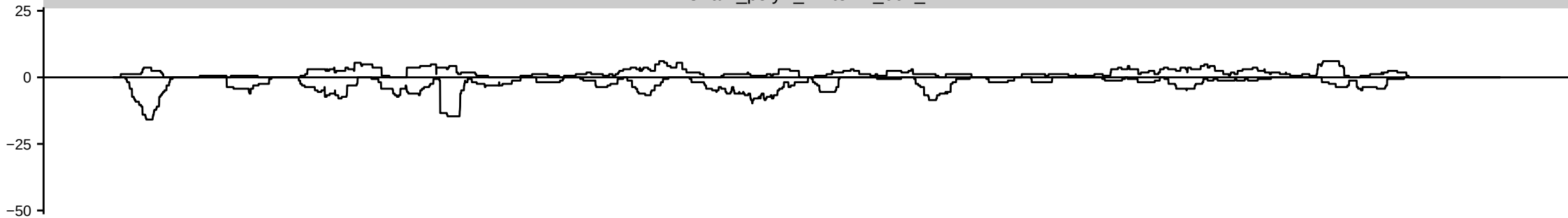
HsBam_polyA_whiteKD_00h_B
