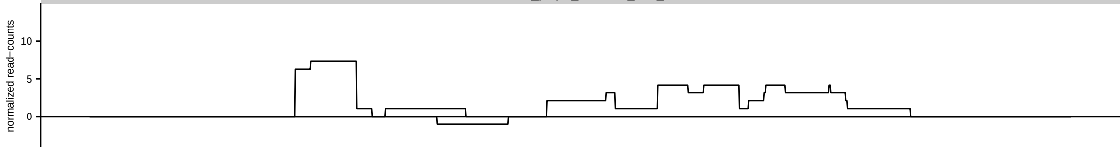
HsBam_polyA_whiteKD_68h_A
