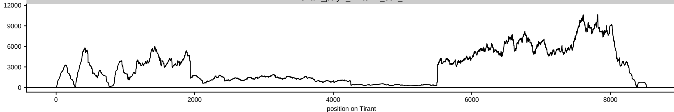
HsBam_polyA_whiteKD_00h_B
