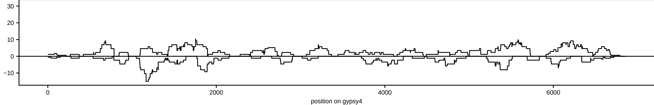
HsBam_polyA_whiteKD_00h_B
