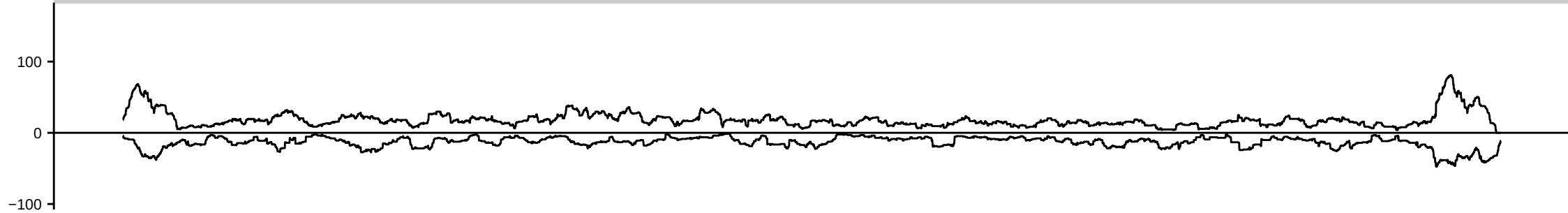
HsBam_polyA_whiteKD_42h_B
