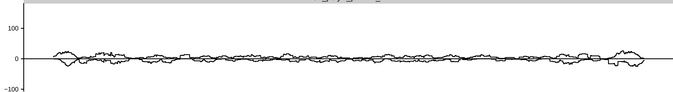
OV_polyA_piwiKD_B
