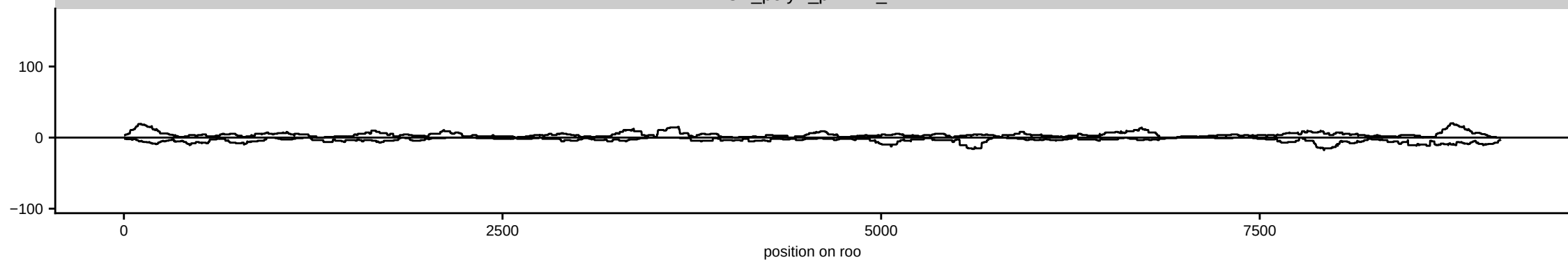
OV_polyA_piwiKD_B
