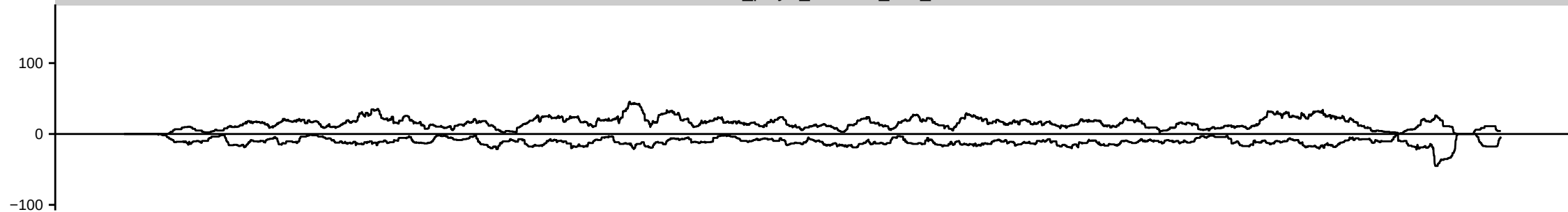
HsBam_polyA_whiteKD_00h_B
