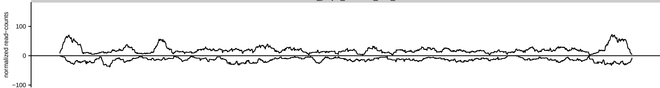
HsBam_polyA_whiteKD_68h_A
