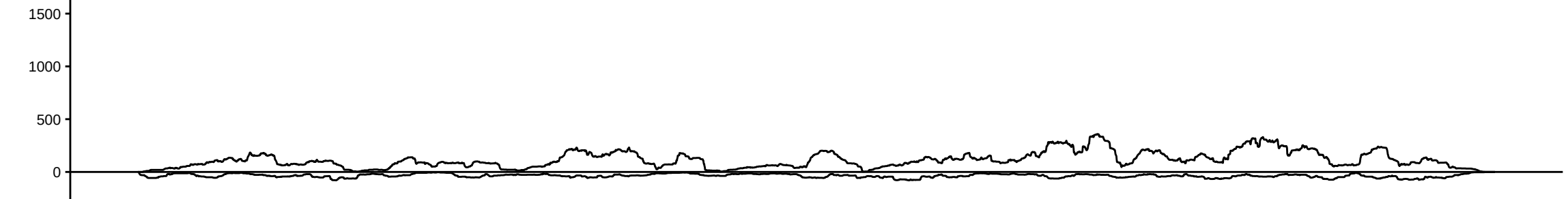
TosK_PiwiAub_X
