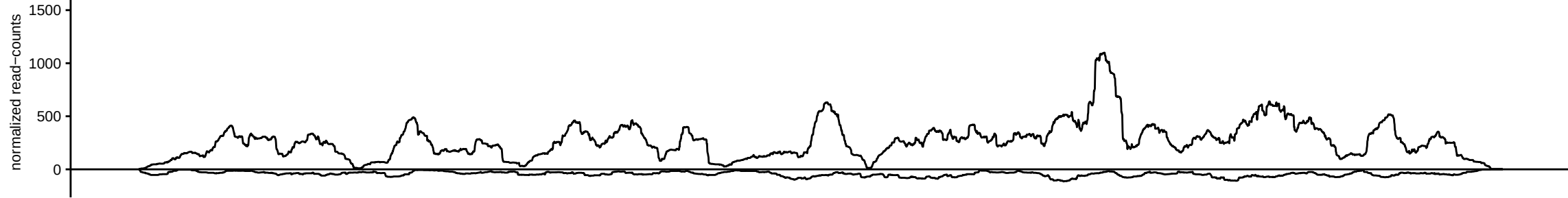
MTD_AubAgo3_C
