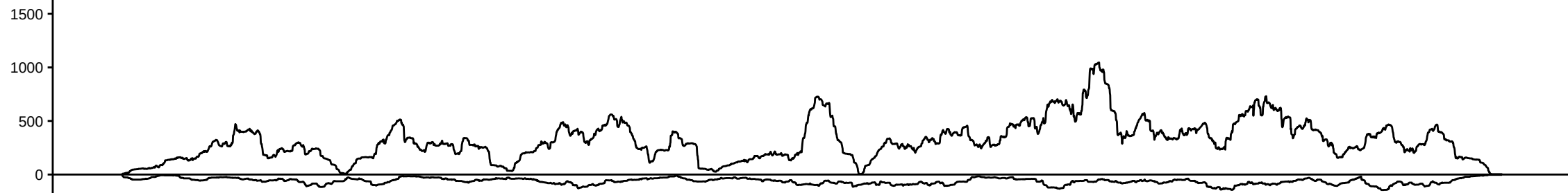
TOSK_AubAgo3_B
