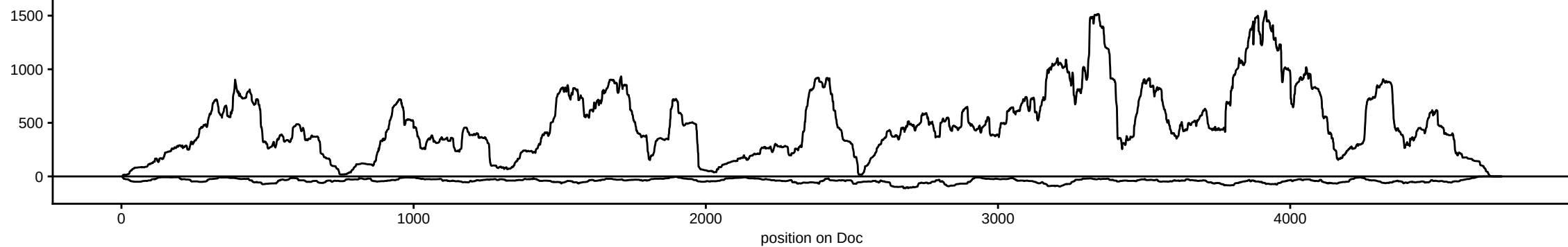
TOSK_AubAgo3_C
