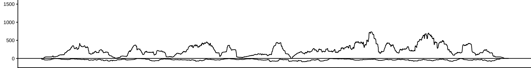
MTD_AubAgo3_C
