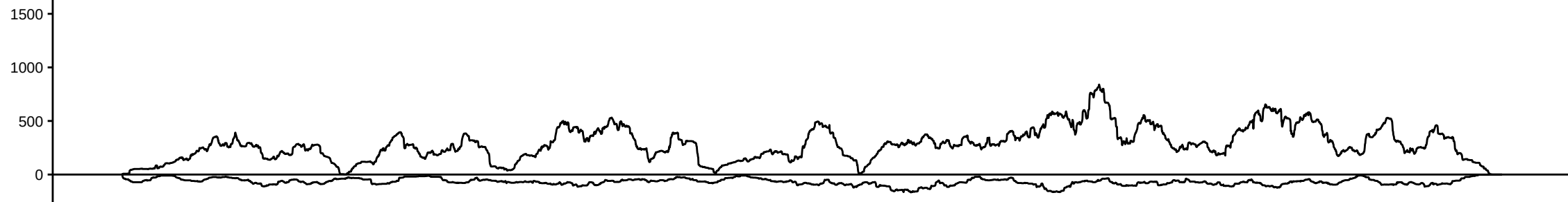
MTD_AubAgo3_B
