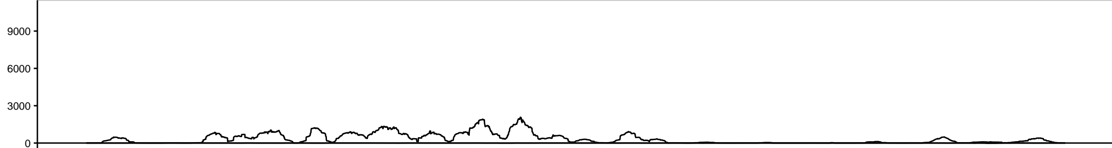
MTD_AubAgo3_C
