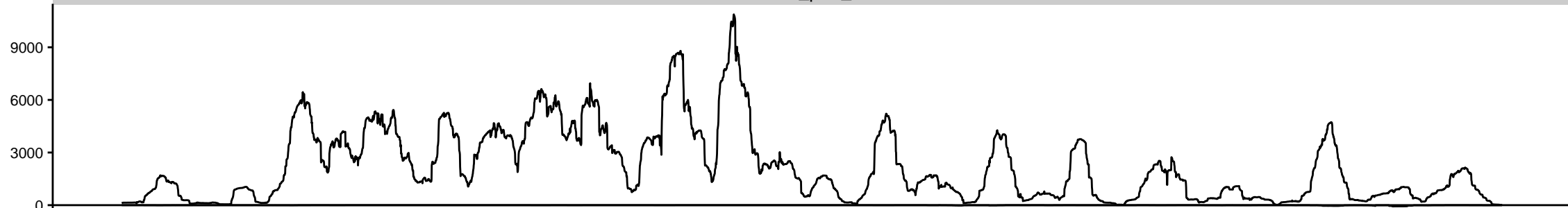
MTD_piwi_C
