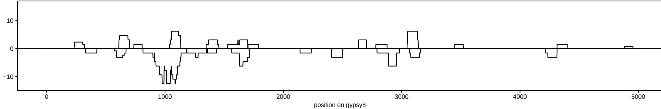
MTD_AubAgo3_C
